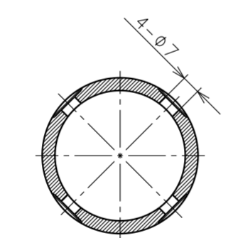
剖视图 A-A (1:2)
