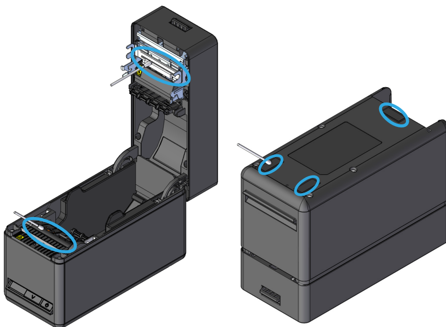
Abbildung 13-1 Reinigen von Thermokopf/Druckwalze/Gummifüßen
