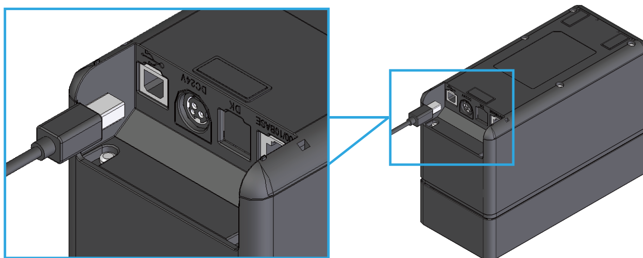
Abbildung 12-1 Verbindung von USB-Kabel
